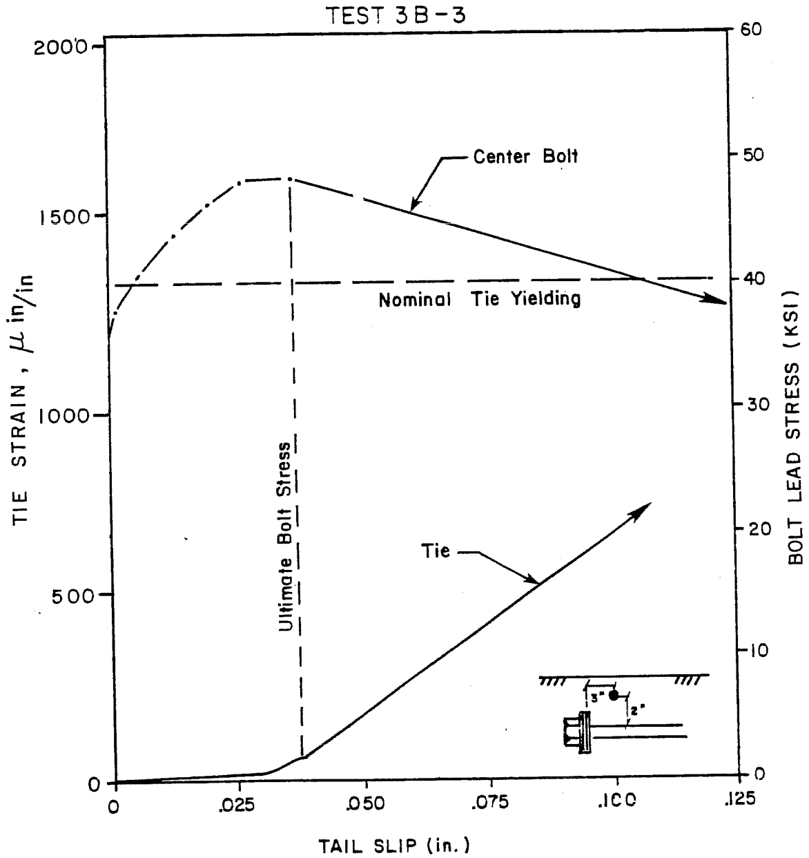
Fig. 4.27 Tie strains, 3B-3
